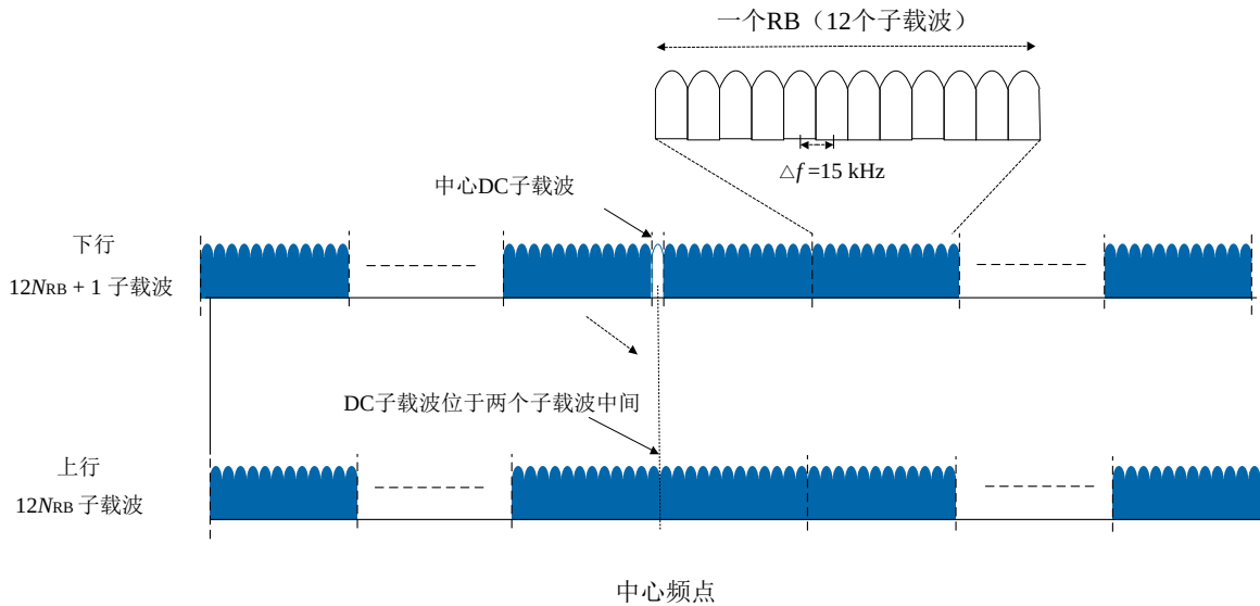
图1 直流子载波的位置
