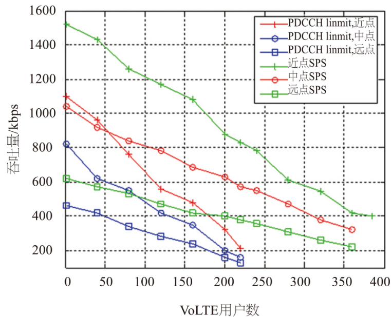
图2 VoLTE用户数和吞吐量关系
